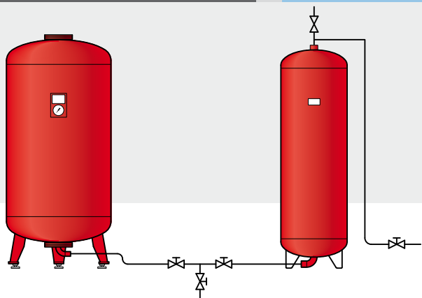
A Flexcon előtét tartály csatlakoztatása
